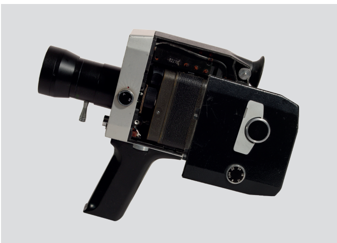
Camera KMZ « Quartz » 1x8 S-2 modifiée par le KGB (URSS), avec un appareil photo F-22 « NAILON » caché à l'intérieur et permettant la prise de photo clandestine à un angle de 90°. Movie camera KMZ "Quartz" 1x8 S-2 modified by the KGB (USSR), with camera F-22 "NAILON" hidden inside and allowing the taking of clandestine photos at an angle of 90°.
